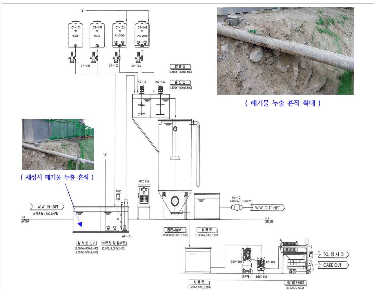
[그림] 오폐수 처리시설 배치도 및 누출 상태
